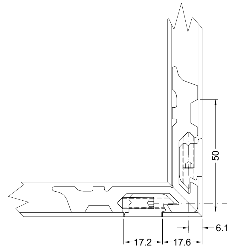
COUPE B-B
